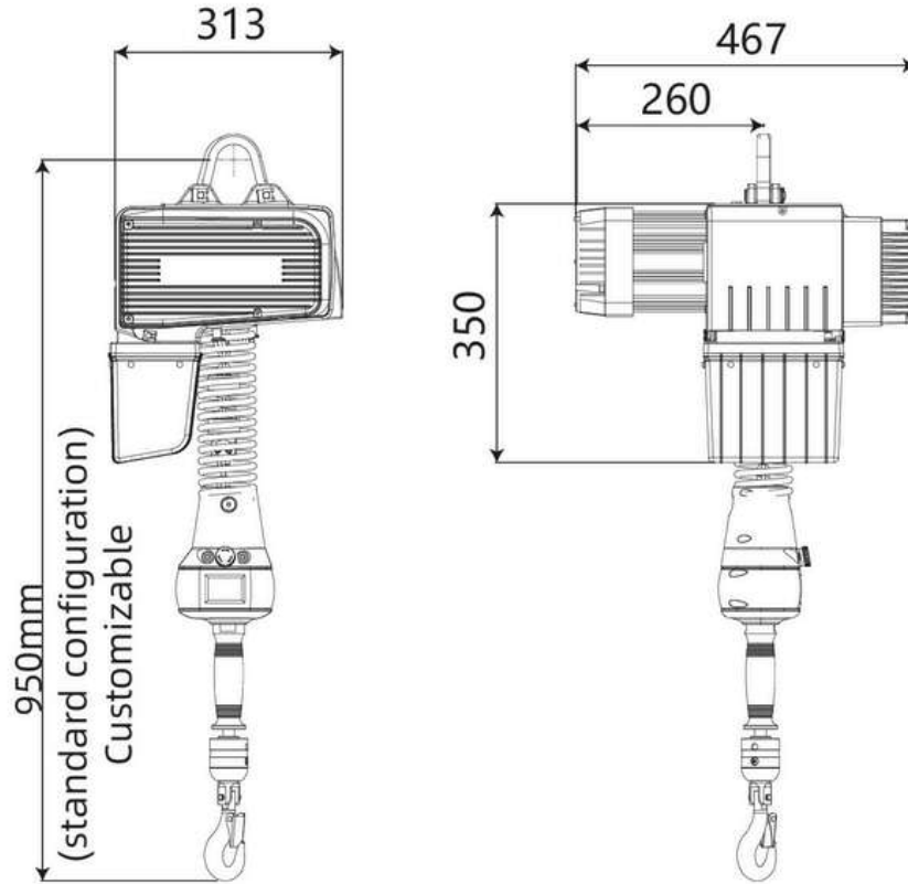
ST12-500 Serisi Ürün Boyutu
