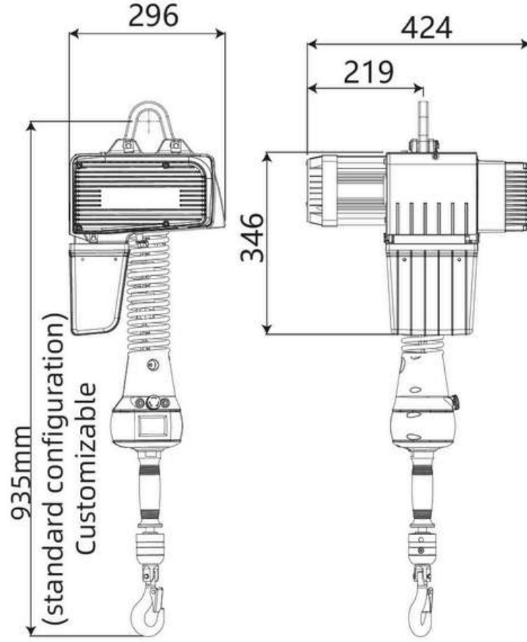
ST12-125/ST12-250 Serisi Ürün Boyutu
